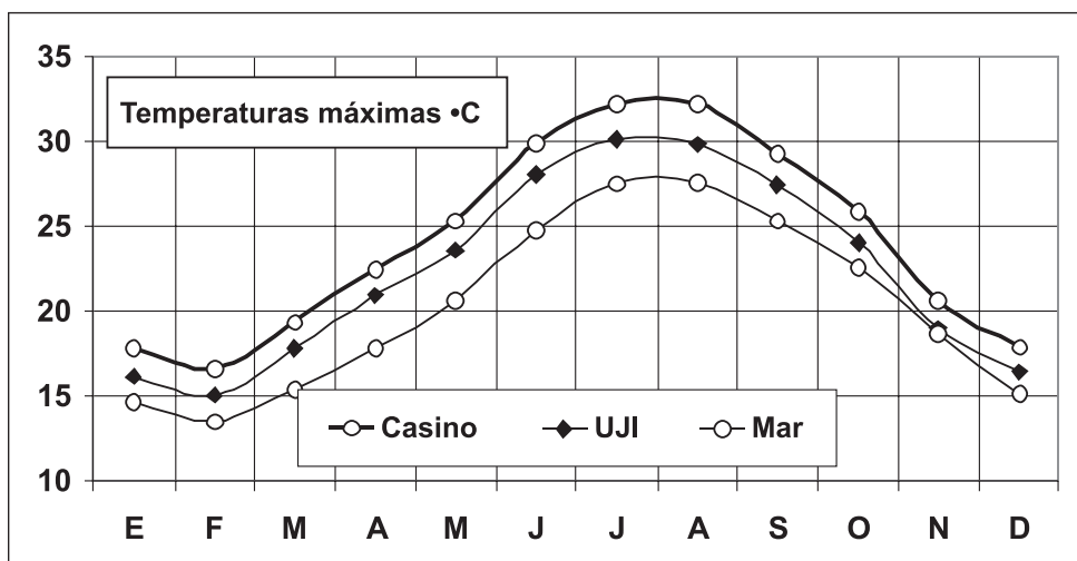
FIGURA 10. Régimen anual de las temperaturas máximas.
