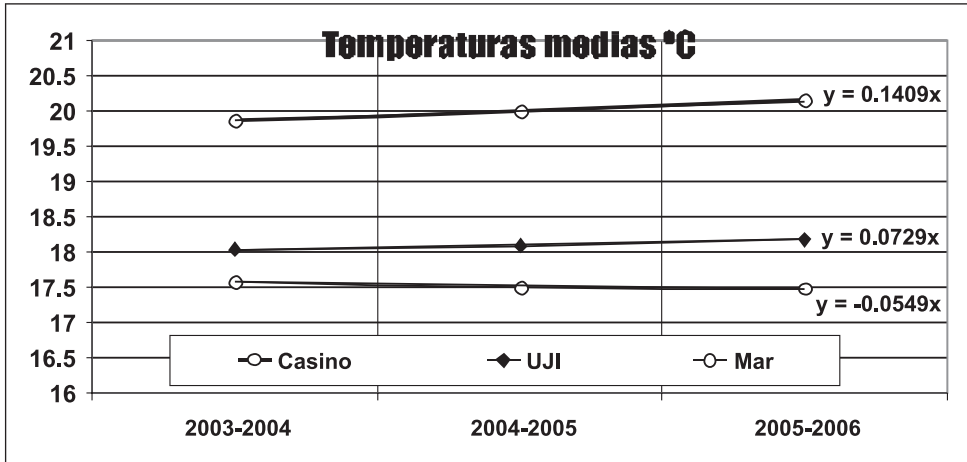
FIGURA 8. Evolución de la temperatura media anual.
