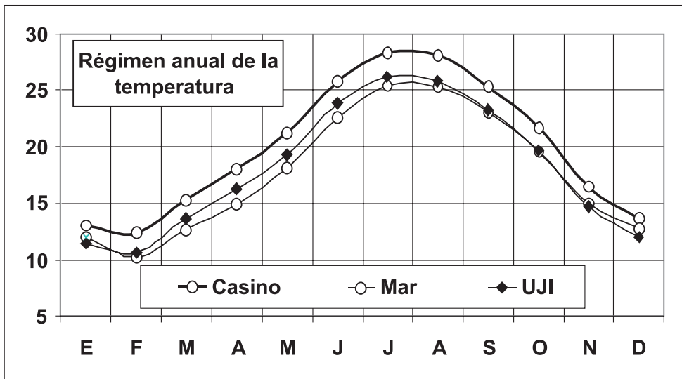
FIGURA 9. Régimen anual de la temperatura.
