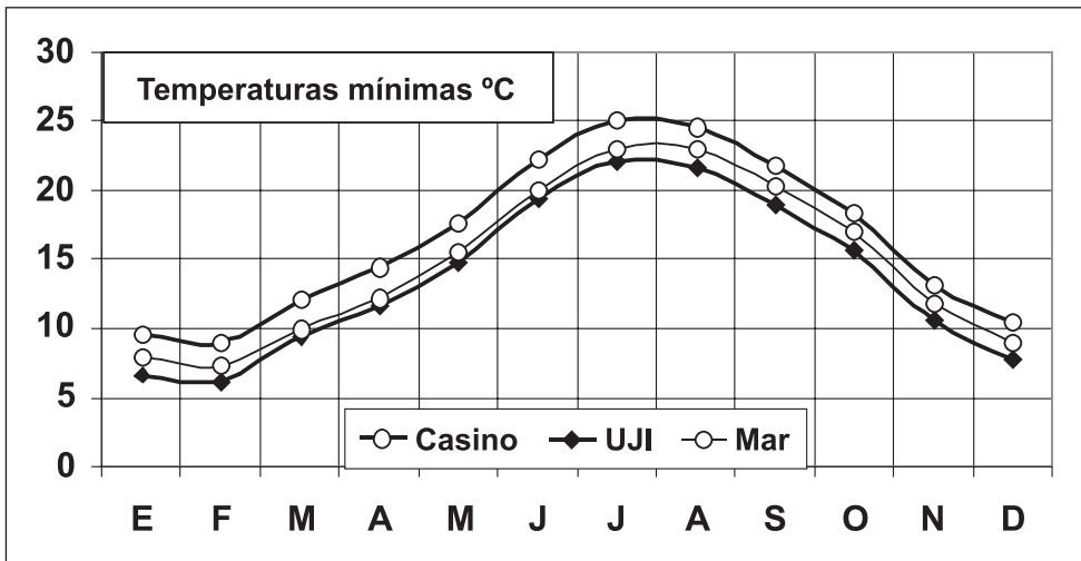
FIGURA 12. Régimen anual de las temperaturas mínimas.
